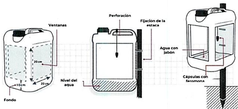
Figura 1. Elaboración e instalación de trampas tipo bidón. Créditos: INIFAP, 2017.
